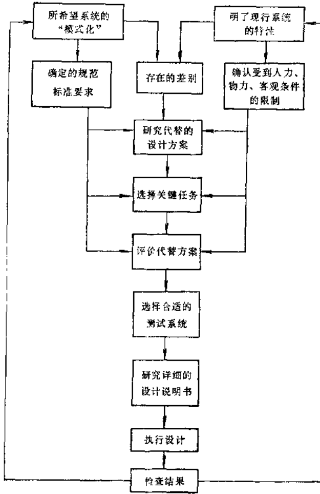
图1-1-3 测试系统设计程序
