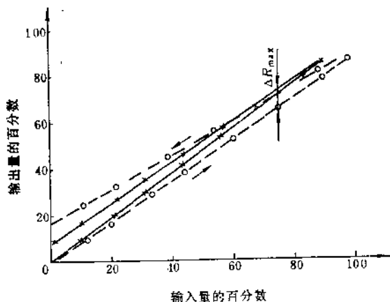
图1-3-4 重复性
