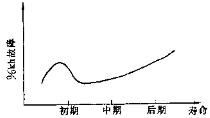
图1-2-27 %故障率与寿命的关系 对于元件故障,可在静态下进行测试,也就是
