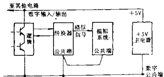
图1-3-24 使模拟和数字地线间的阻抗最小的接法
