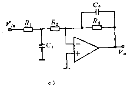
图1-3-29 简单的RC有源低通滤波器
