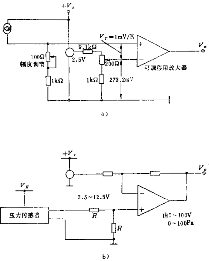
图1-3-68 量程偏置
