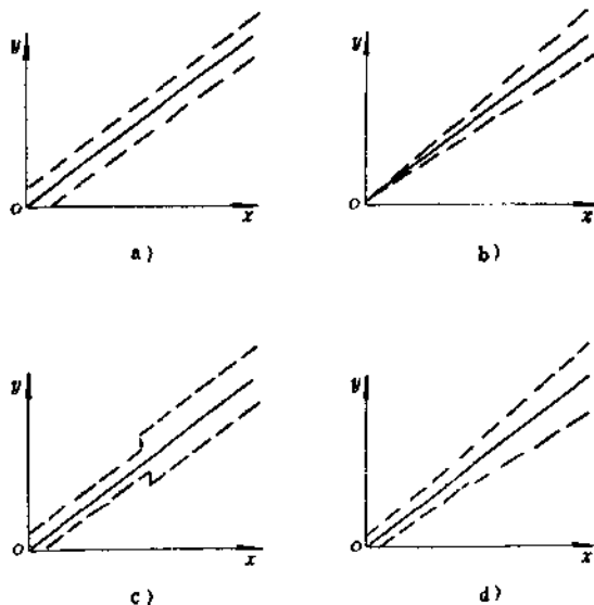
图1-3-7 几种误差带
